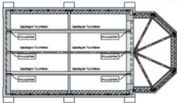
Dakconstructie
