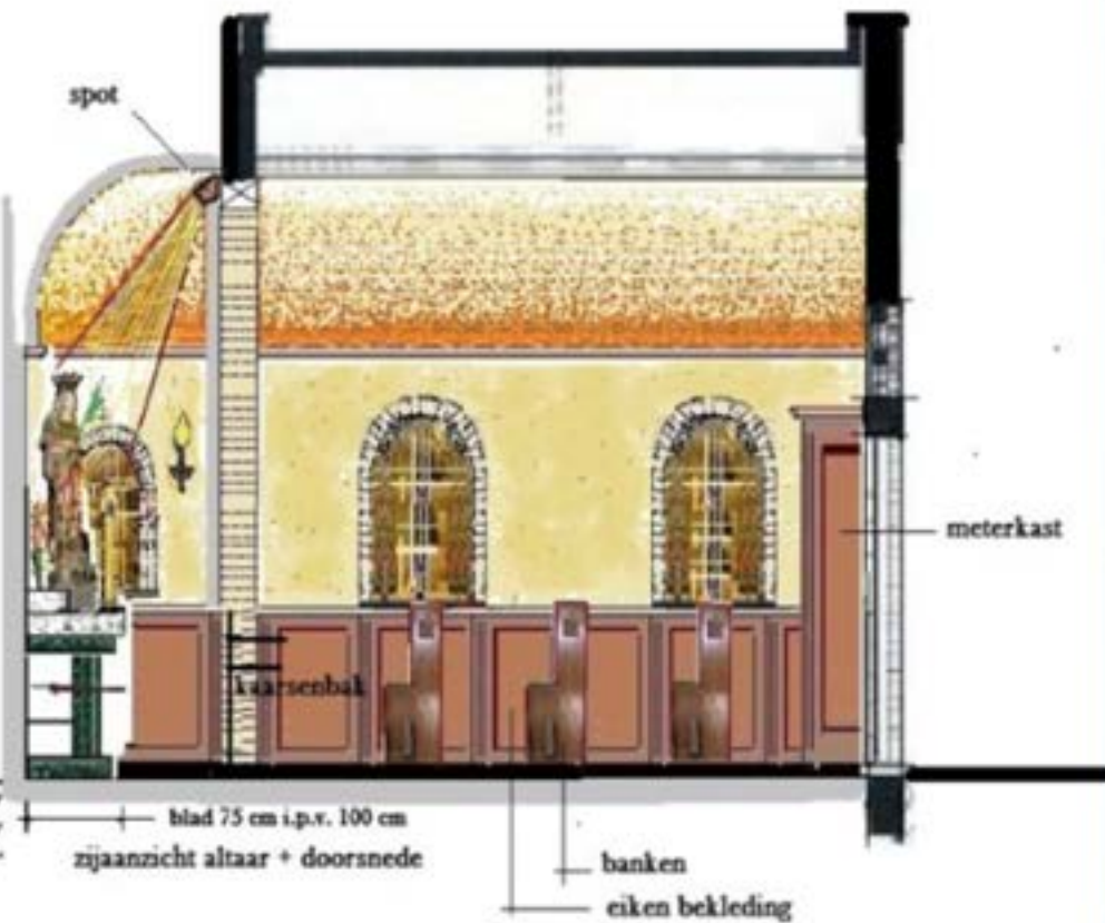
Aanzicht lengte doorsnede
