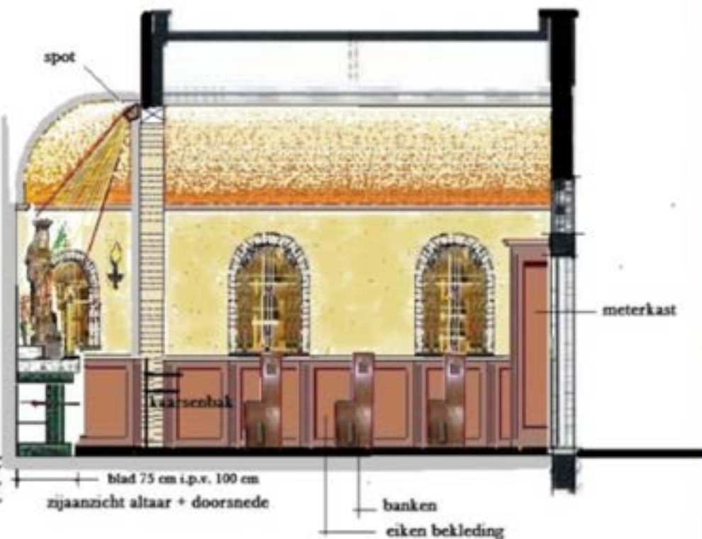
Aanzicht lengte doorsnede
