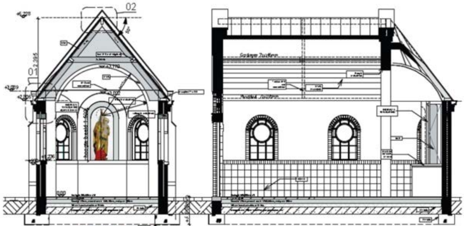
SNEDE AA
