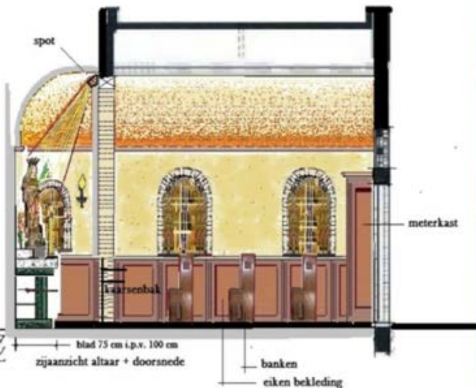
Aanzicht lengte doorsnede
